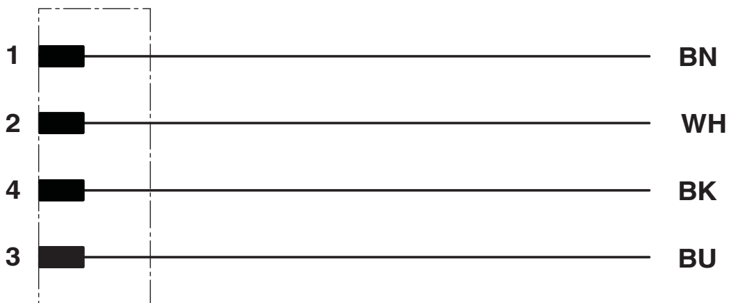
Equipaggiamento dei contatti del connettore M12
