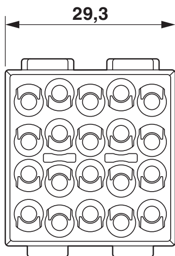
Insero portacontatti femmina
