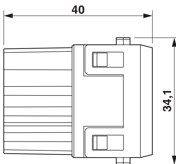
Disegno quotato
