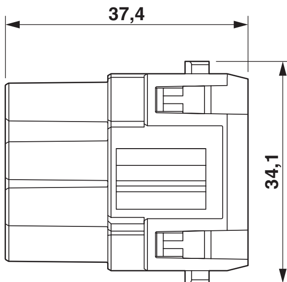
Disegno quotato
