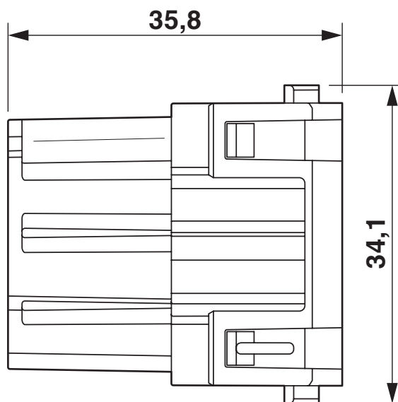
Disegno quotato
