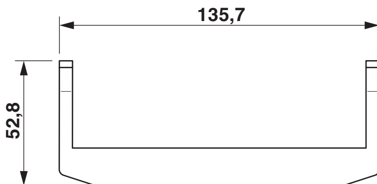
Disegno quotato
