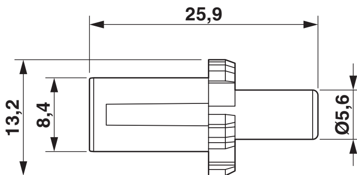
Disegno quotato
