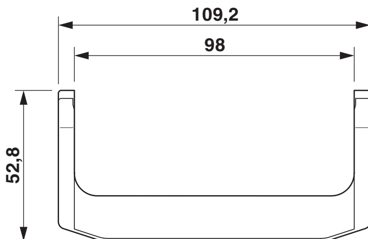
Disegno quotato
