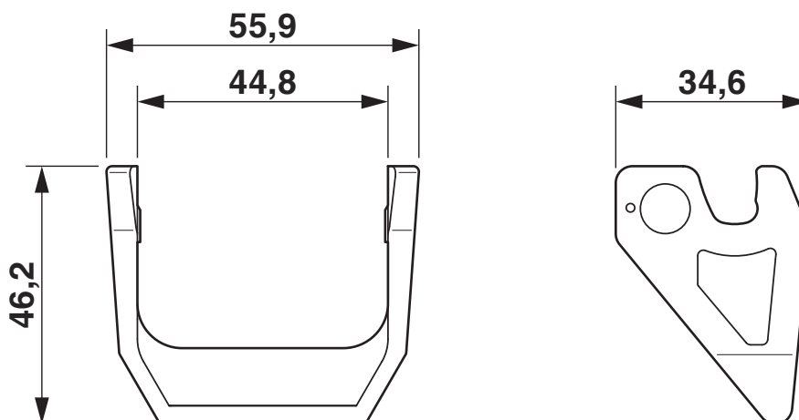
Disegno quotato
