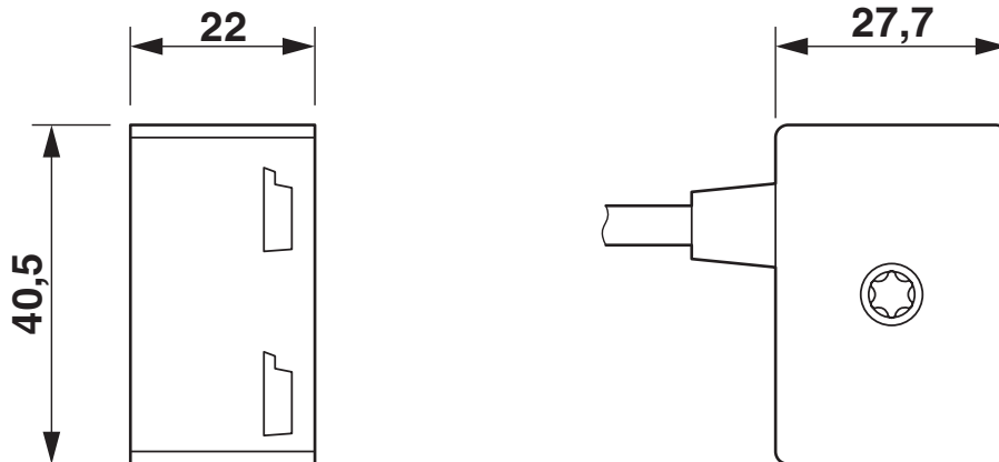
Disegno quotato
