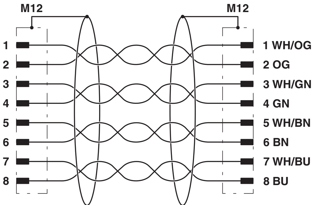
Equipaggiamento dei contatti del connettore M12
