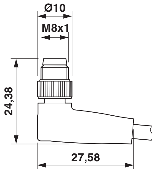
Disegno quotato
