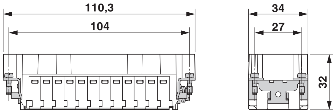
Disegno quotato
