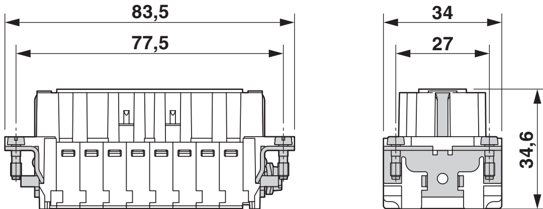
Disegno quotato
