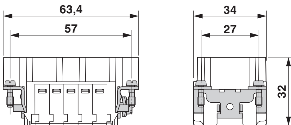
Disegno quotato
