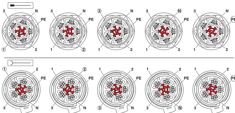
Disegno funzionamento
