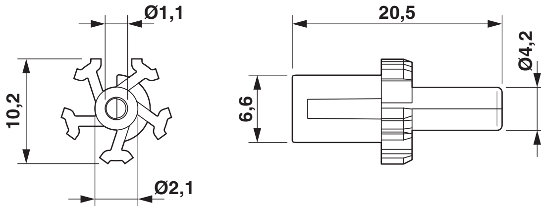
Disegno quotato
