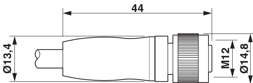
Disegno quotato
