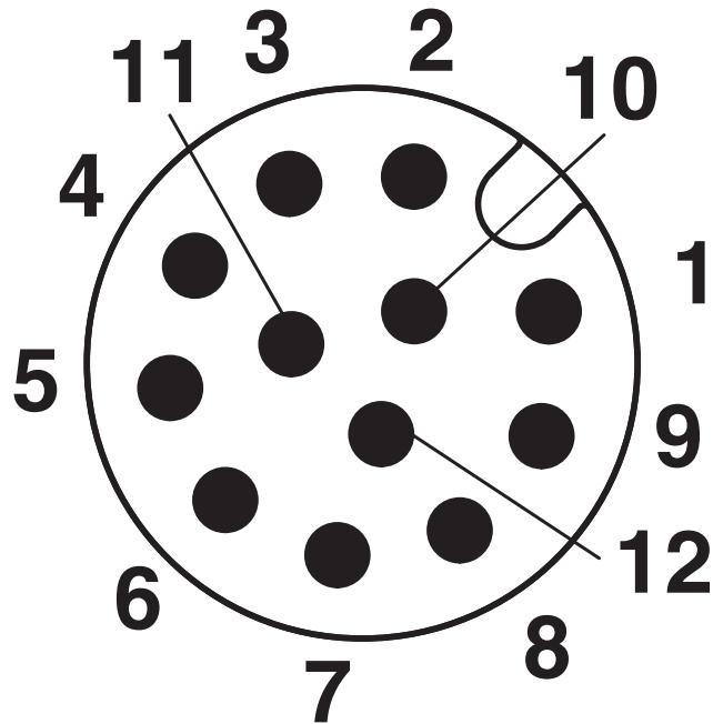
Disegno schema
