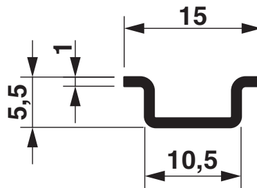
Disegno quotato
