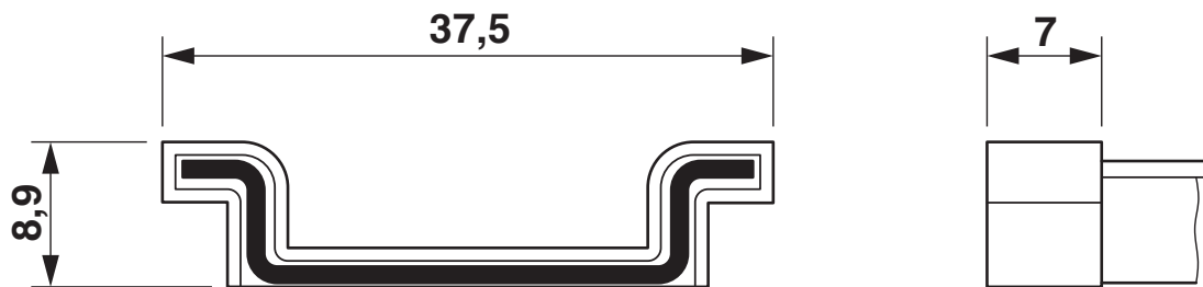
Disegno quotato
