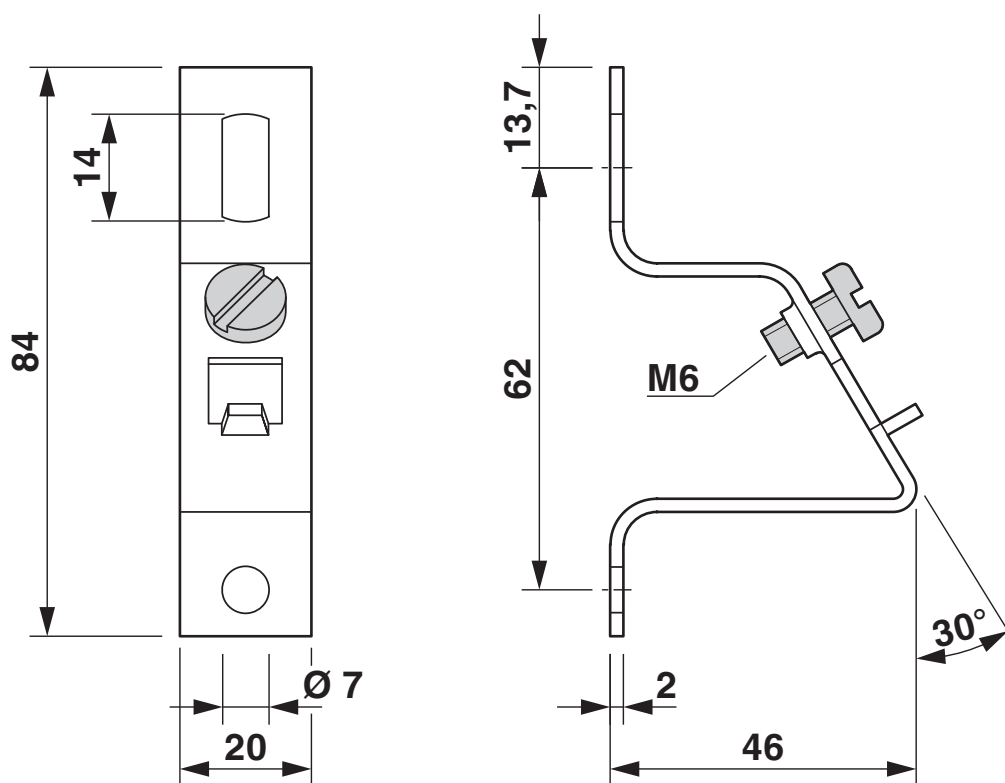
Disegno quotato
