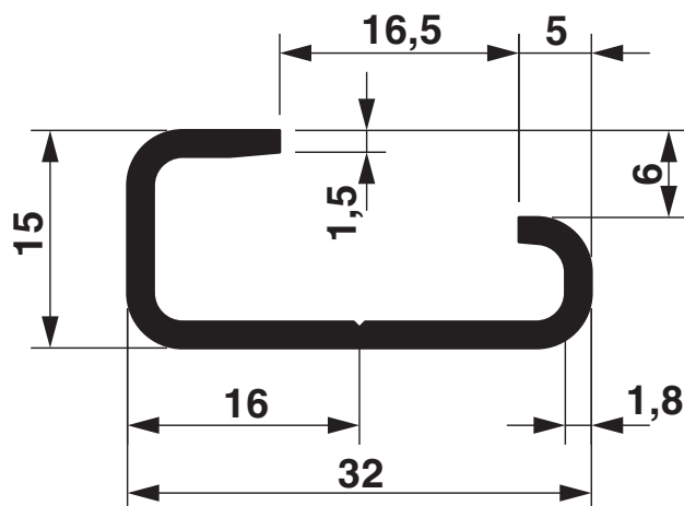
Disegno quotato
