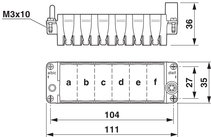
Disegno quotato
