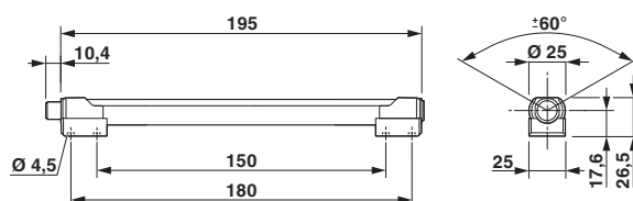
Disegno quotato
