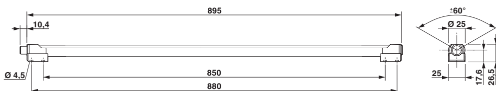
Disegno quotato
