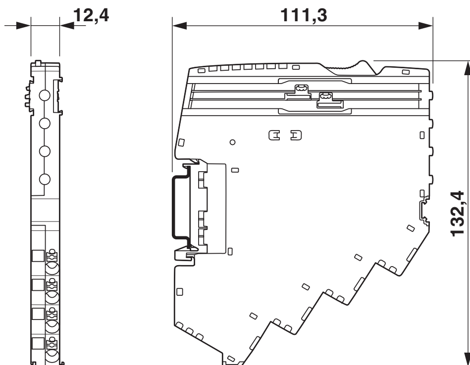
Disegno quotato
