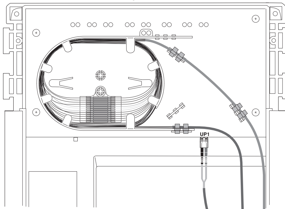
Disegno schema
