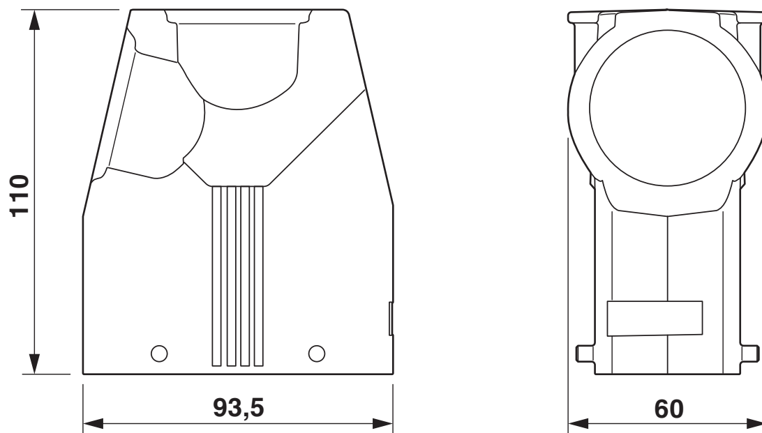
Disegno quotato
