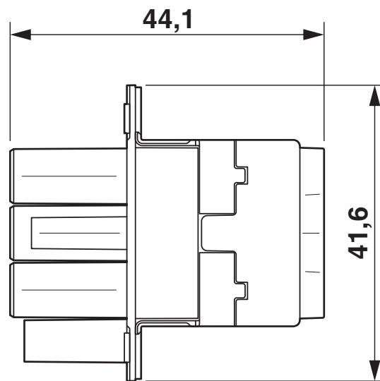
Disegno quotato
