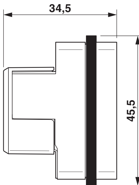
Disegno quotato
