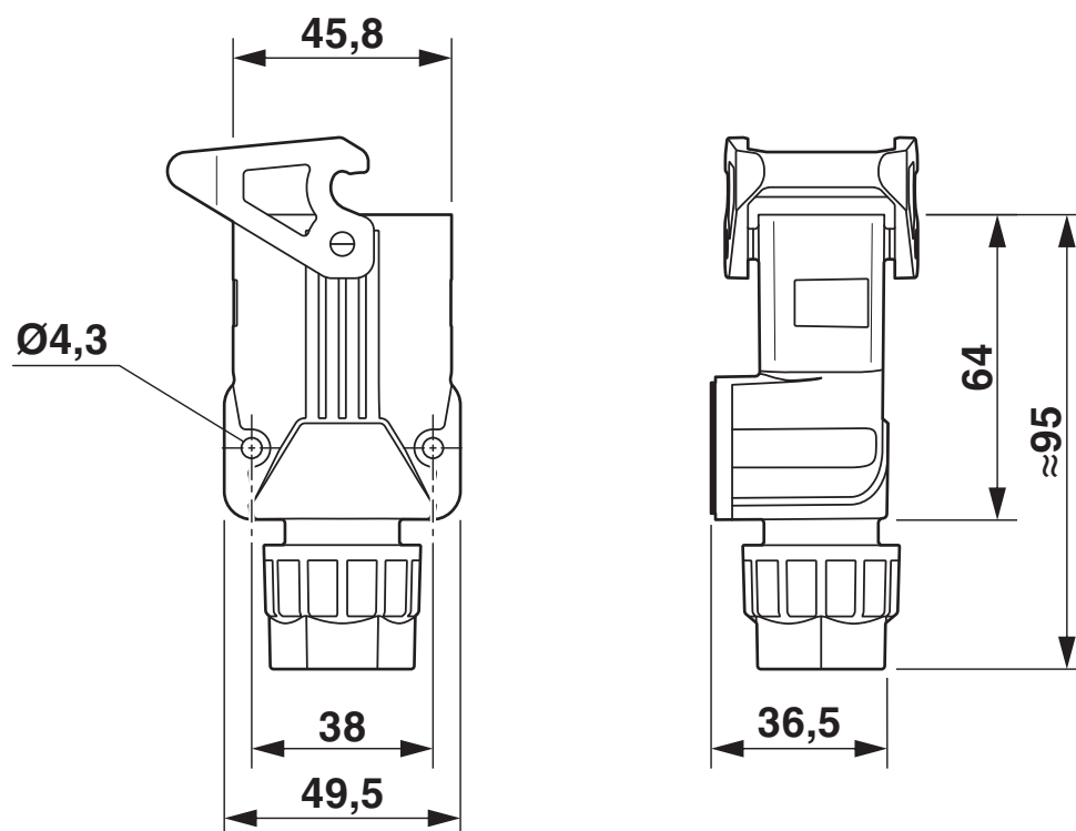
Disegno quotato
