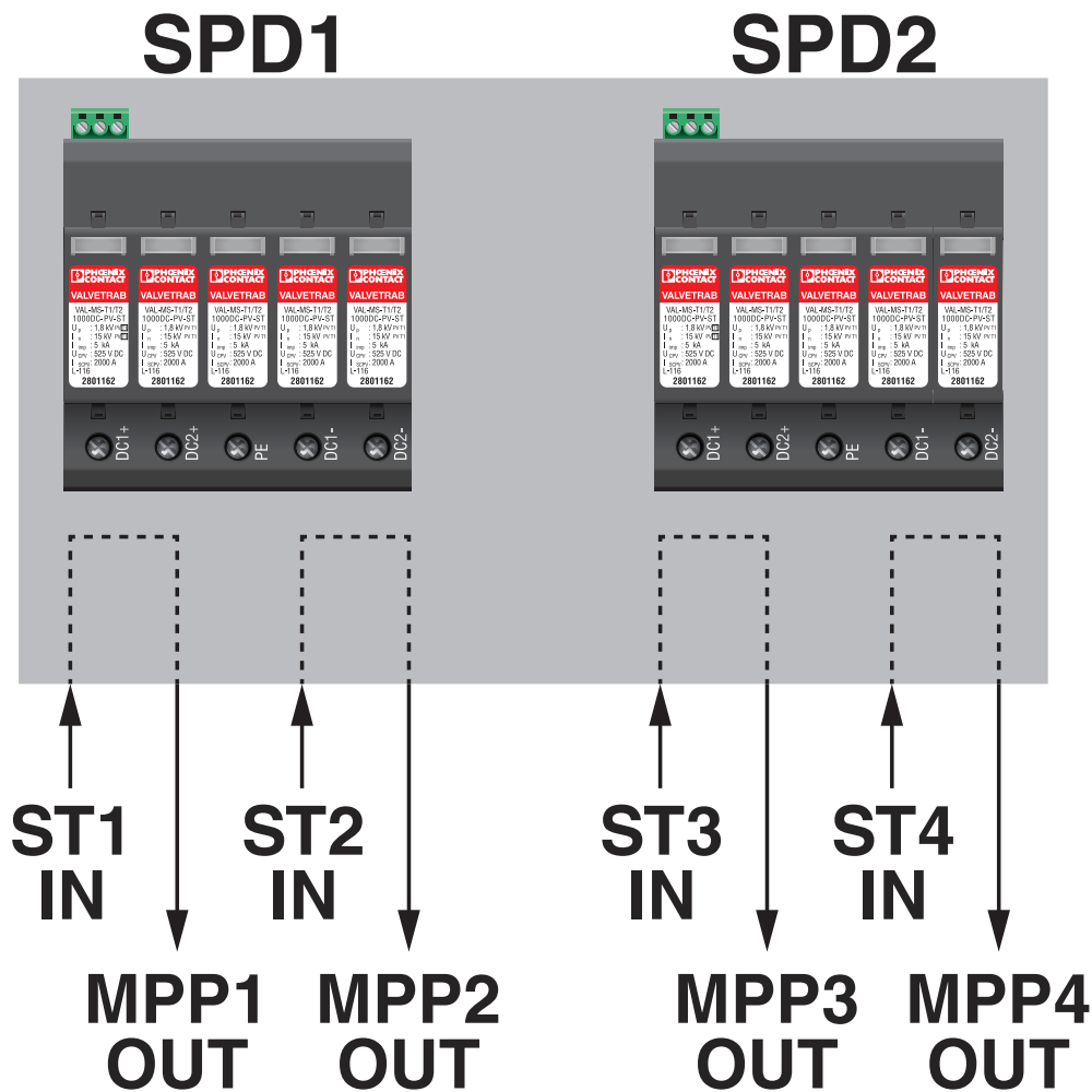
Disegno collegamento
