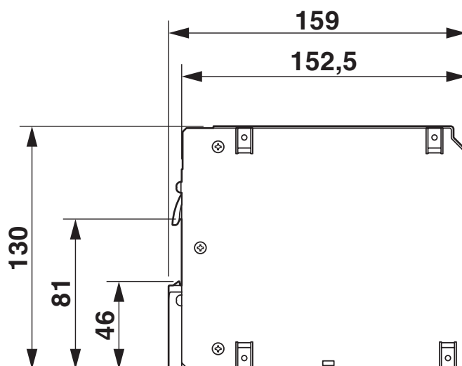
Disegno quotato
