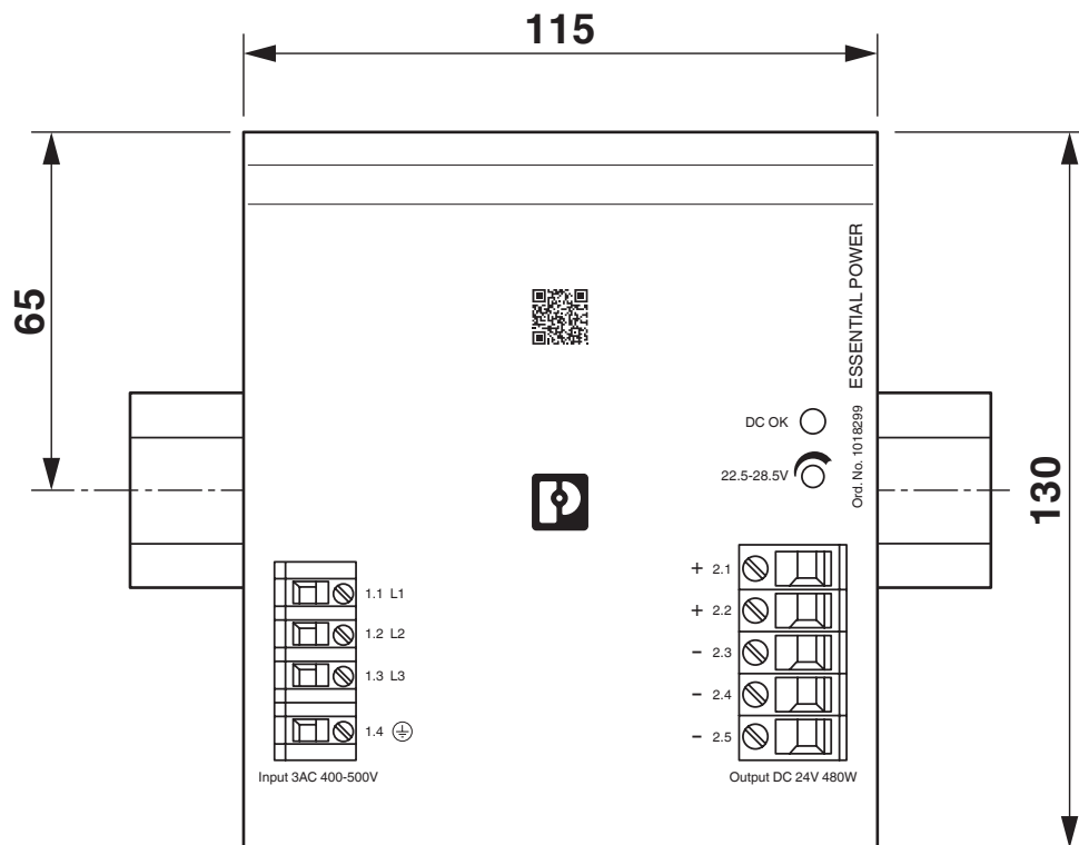
Disegno quotato
