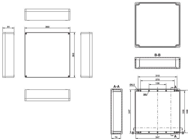
Disegno quotato
