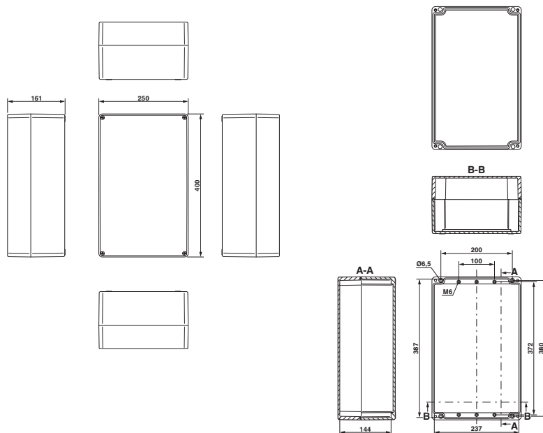
Disegno quotato
