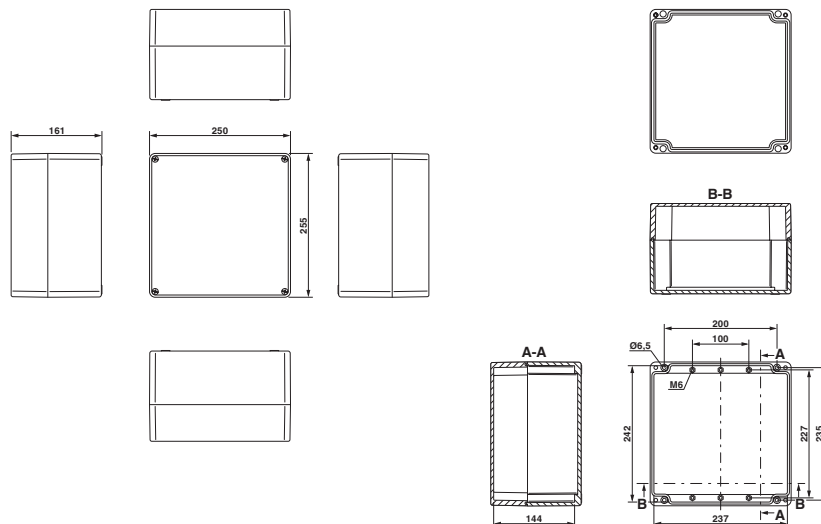
Disegno quotato
