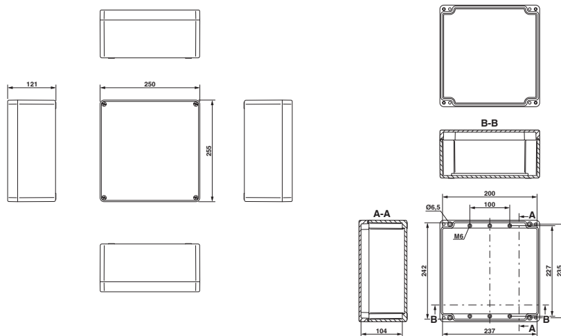
Disegno schema
