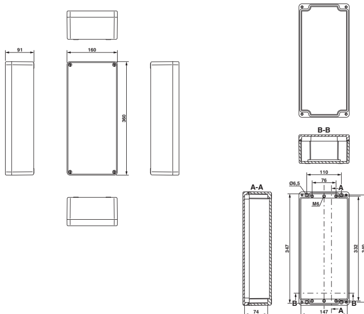
Disegno quotato
