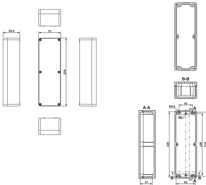
Disegno schema
