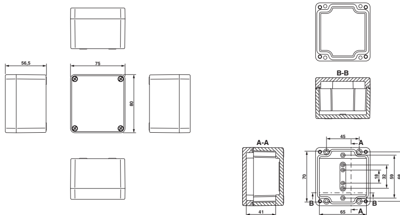
Disegno quotato
