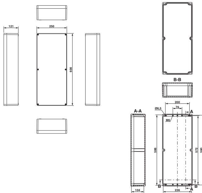
Disegno schema
