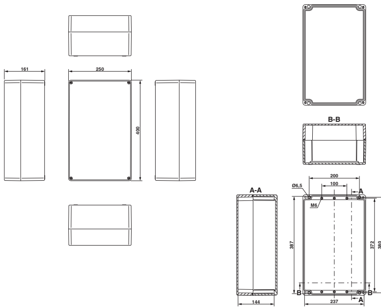
Disegno schema
