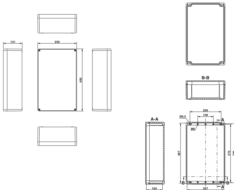
Disegno quotato
