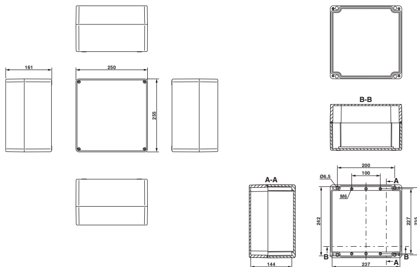
Disegno quotato
