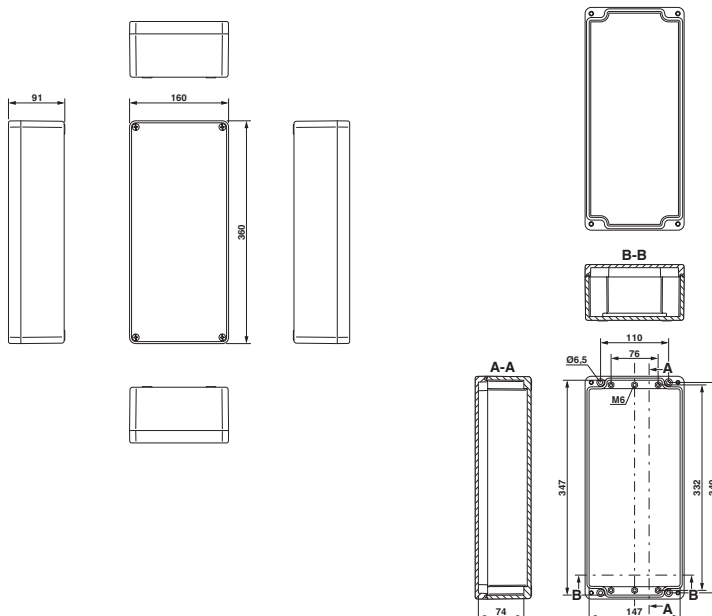
Disegno quotato
