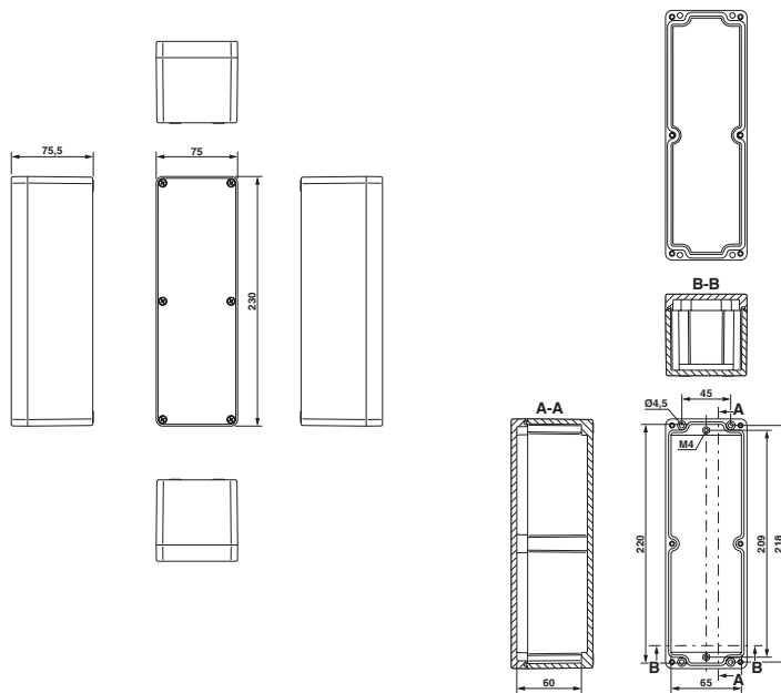
Disegno quotato
