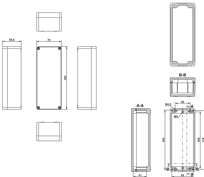
Disegno quotato
