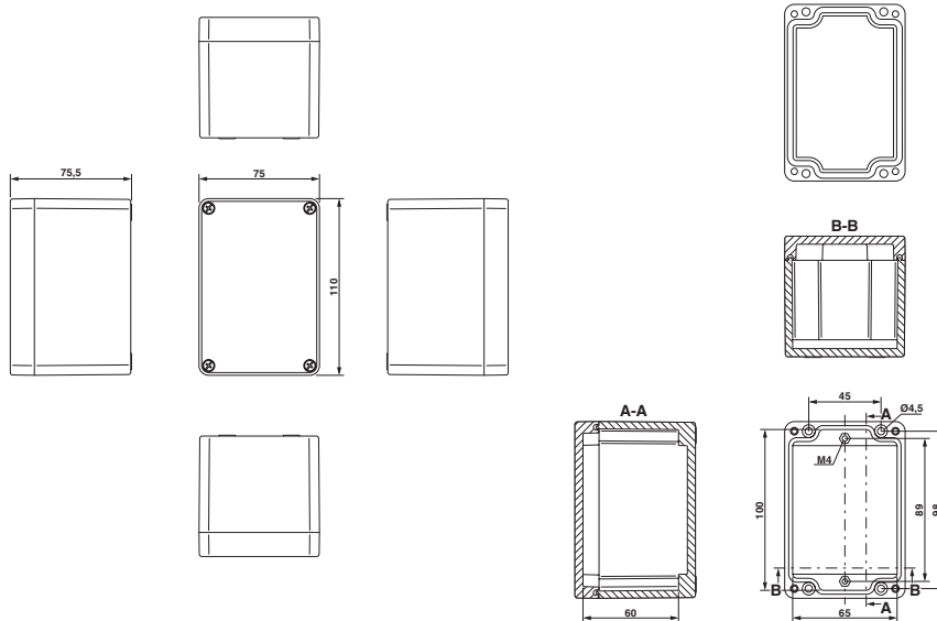
Disegno quotato
