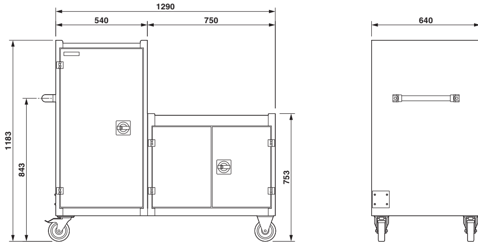
Disegno quotato
