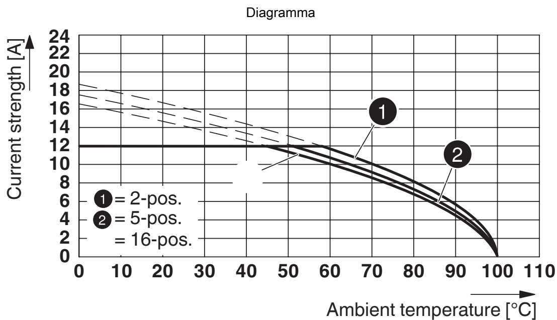
Tipo: SMSTB 2,5/...-STF con DFK-MSTB 2,5/...-GF
