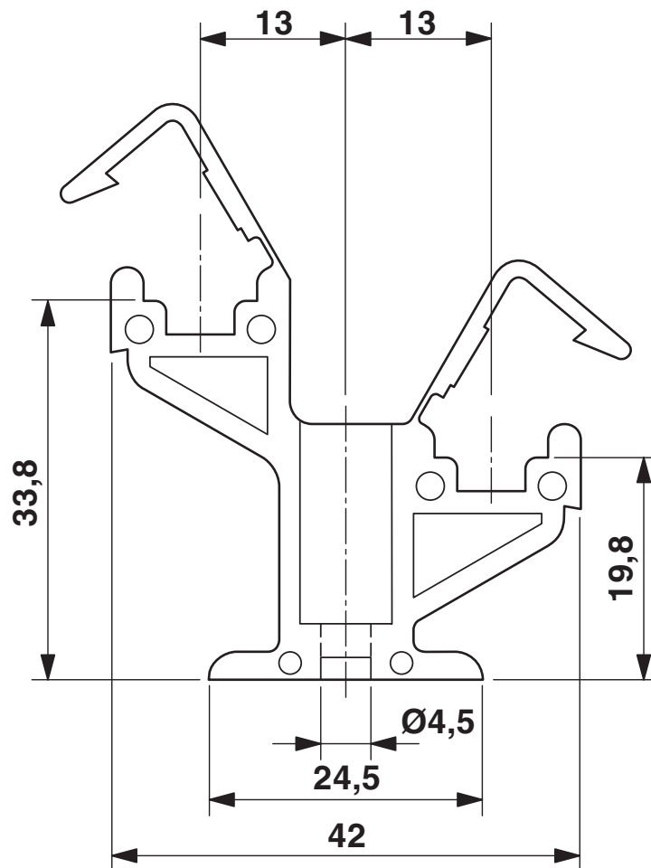
Disegno quotato
